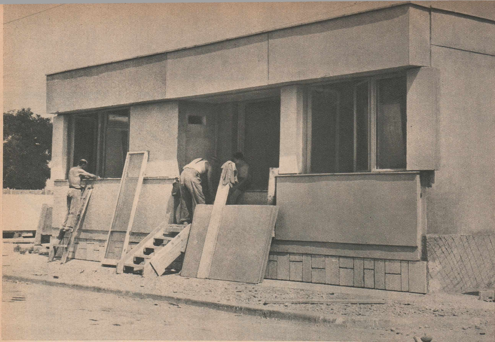
Acest apartament experimental din prefabricate, ridicat în curtea întreprinderii „Progresul” din Capitală, va servi drept model și obiect de studiu pentru constructori.
