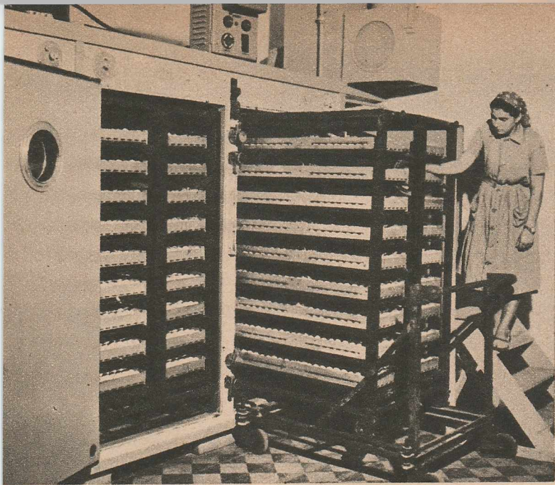
„Mamă” a mii de pui. Controlul ouălor, reglarea temperaturii și a aparatului contribuie la buna desfășurare a cloclirii.
