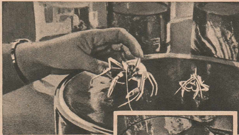
Un crustaceu rar—Munidopsis—un fel de crab care trăiește la peste 4000 de metri adîncime. În dreapta: vietăți pescuite de sovavții sovietici de la Institutul de oceanografie la o adîncime de 8000 de metri sub apele Pacificului.
