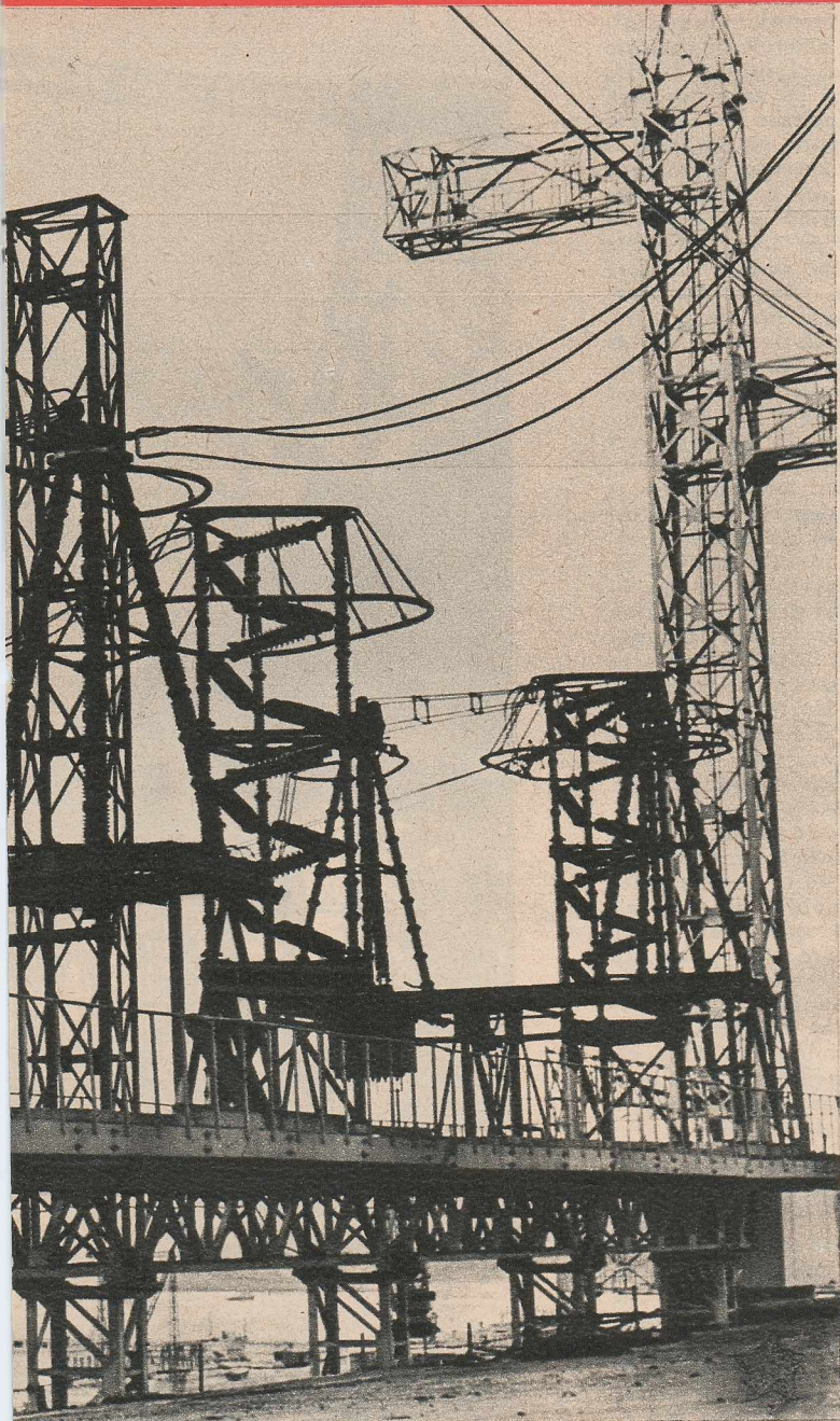
Linie de înaltă tensiune de 500/kV.
