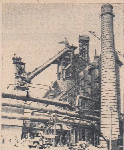
Un furnal nou intrat în funcțiune la uzina metalurgică „V. I. Lenin” din Krivoi Rog.
