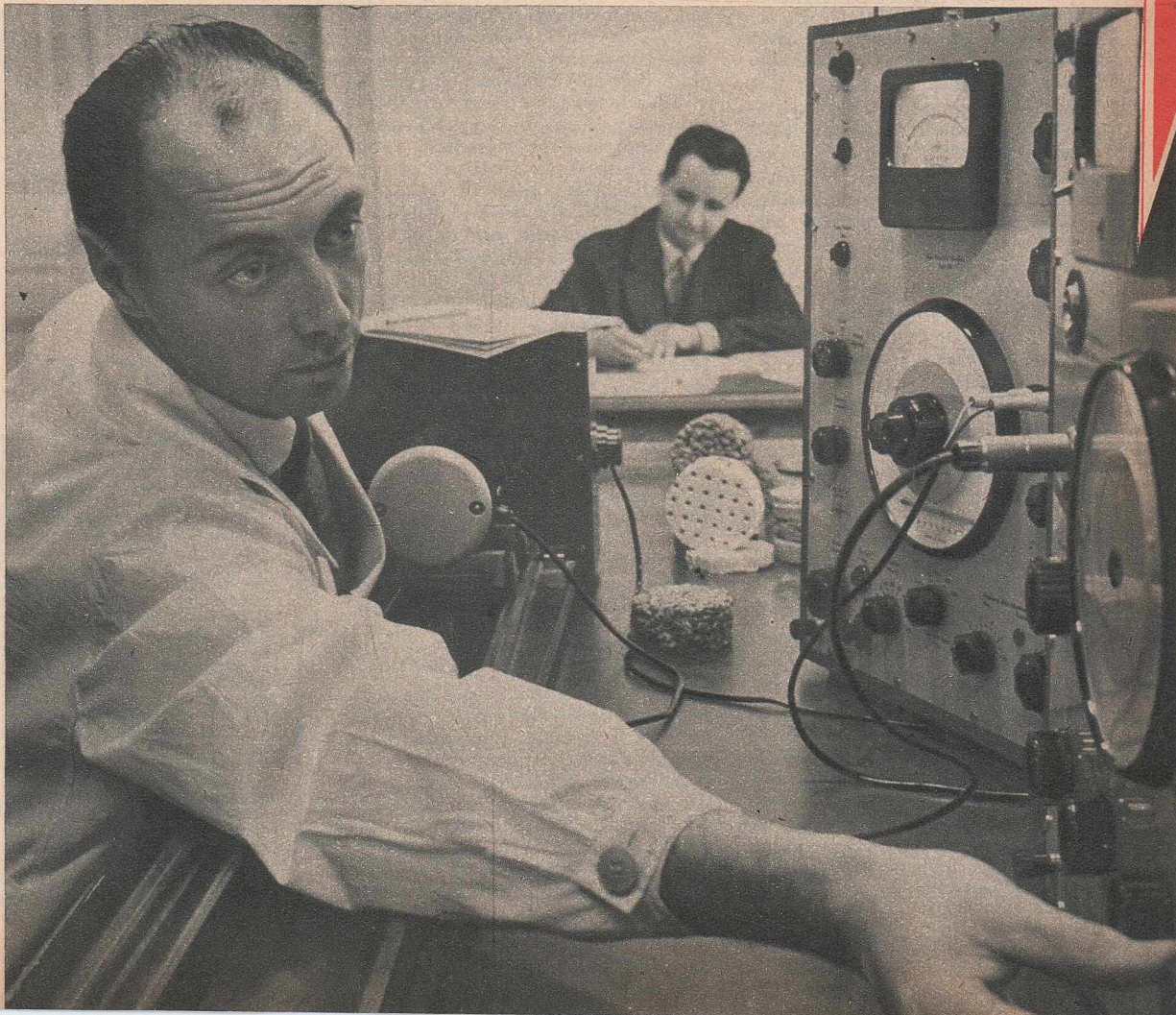
În laboratorul de zgomot industrial al Institutului de protecția muncii sînt măsurate calitățile fono-absorbante ale unor materiale indigene.
