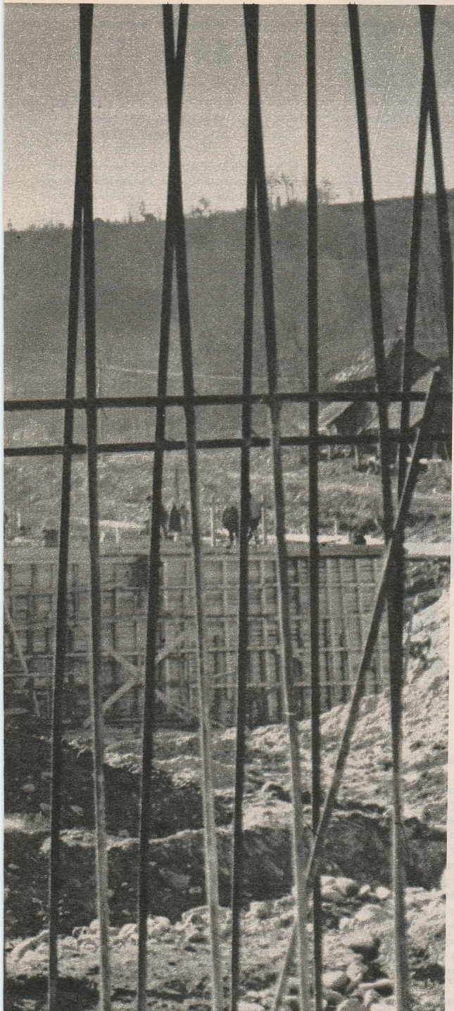
▲ Barajul hidrocentralei Albești II este pregătit pentru betonare. La sfârșitul anului se prevede ca inelul de piatră al barajului să fie apt pentru a reține și distribui după cerințe cei 700 000 mc ai lacului de acumulare.
