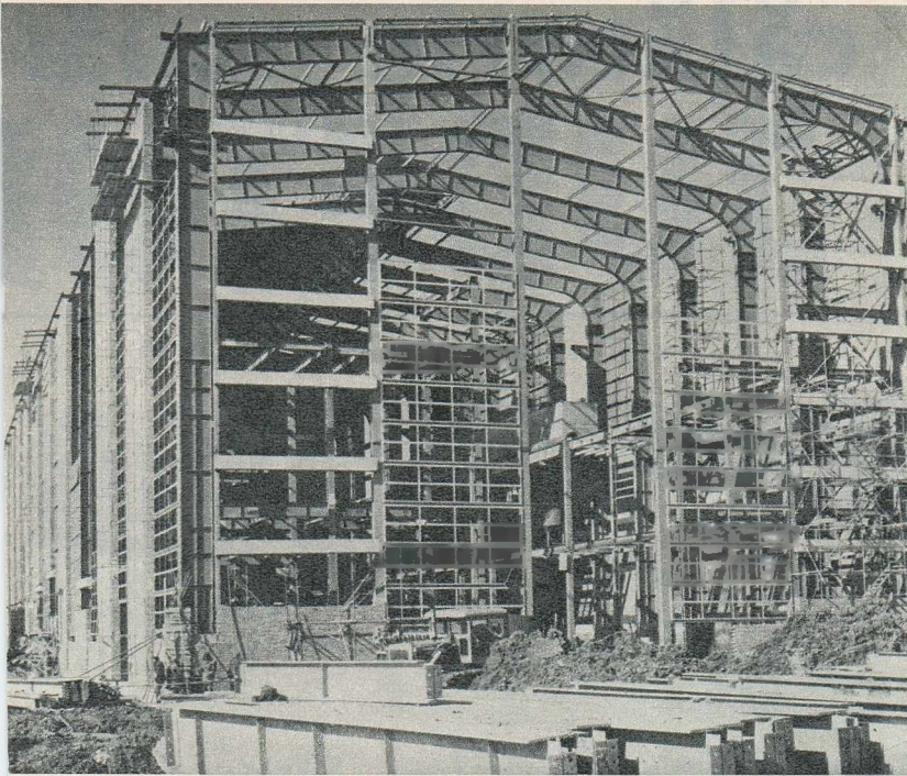
Un aspect de pe șantierul mării fabrici de zahăr ce se construiește acum la Oradea. Construcția reprezintă viitoarea hală de fabricație.
