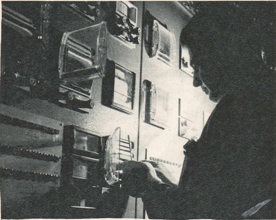
Se verifică tabloul de comandă al secției de polimerizare (Trifu Coman, electrician-șef).
