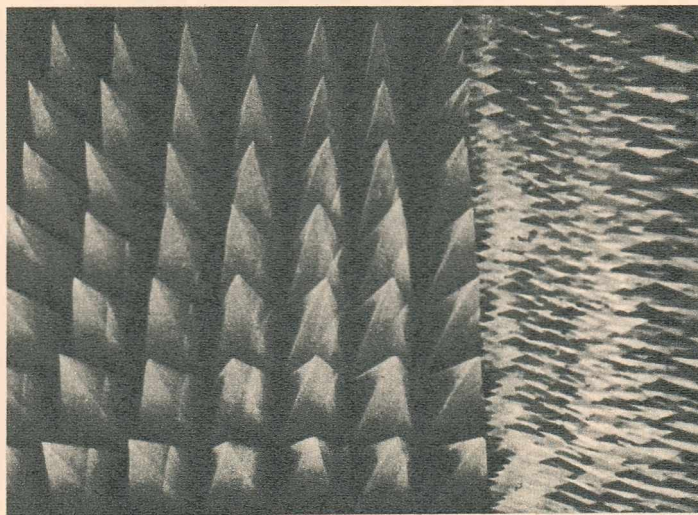
În această încăpere de la centrul spațial de la Houston se efectuează experiențe cu antenele navelor cosmice. Prismele din material plastic absorb ecourile undelor radio.
