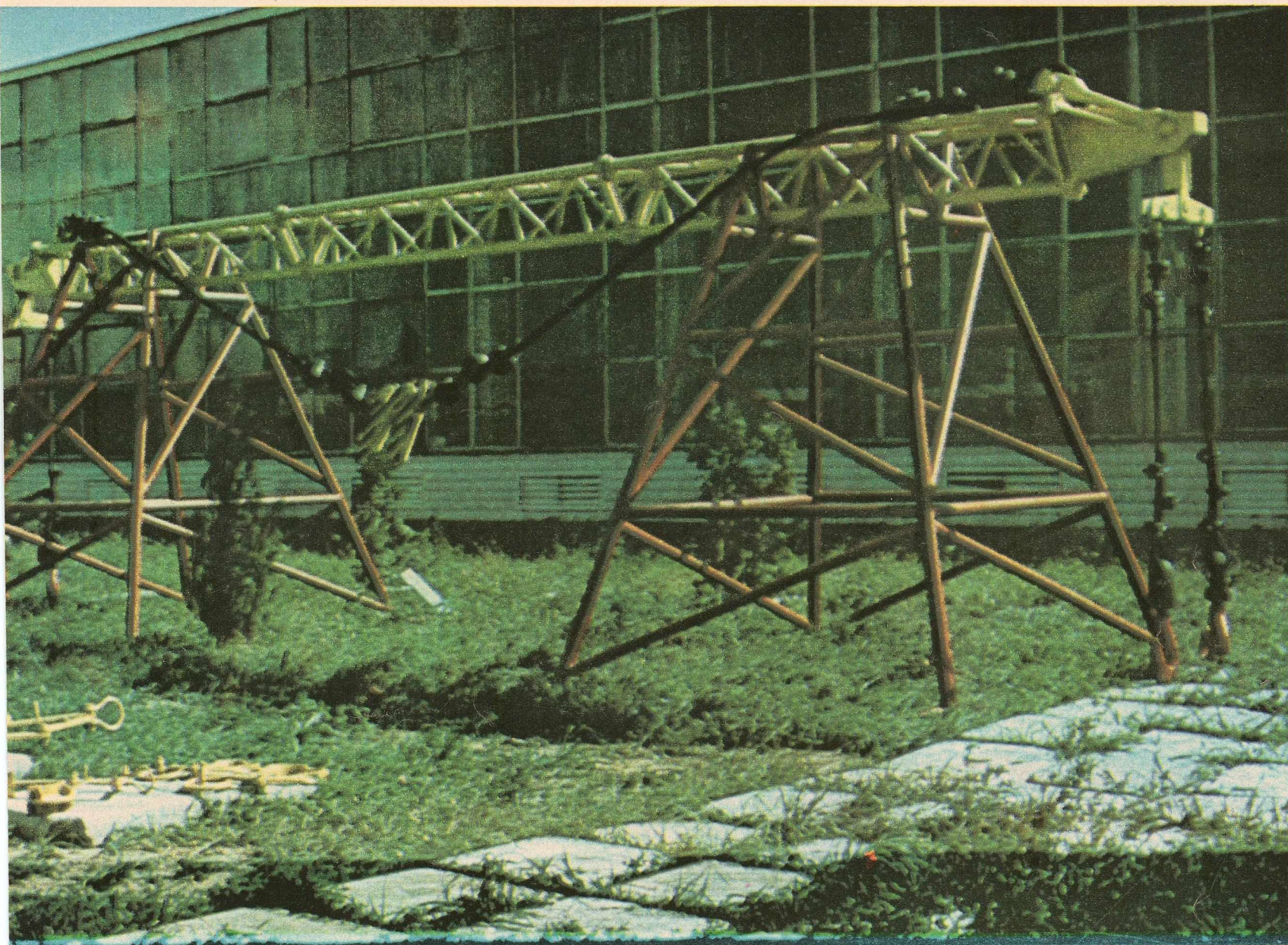
▲ MACARA PORTAL PENTRU DEPOZITE SAU POLIGOANE PREFABRICATE.
