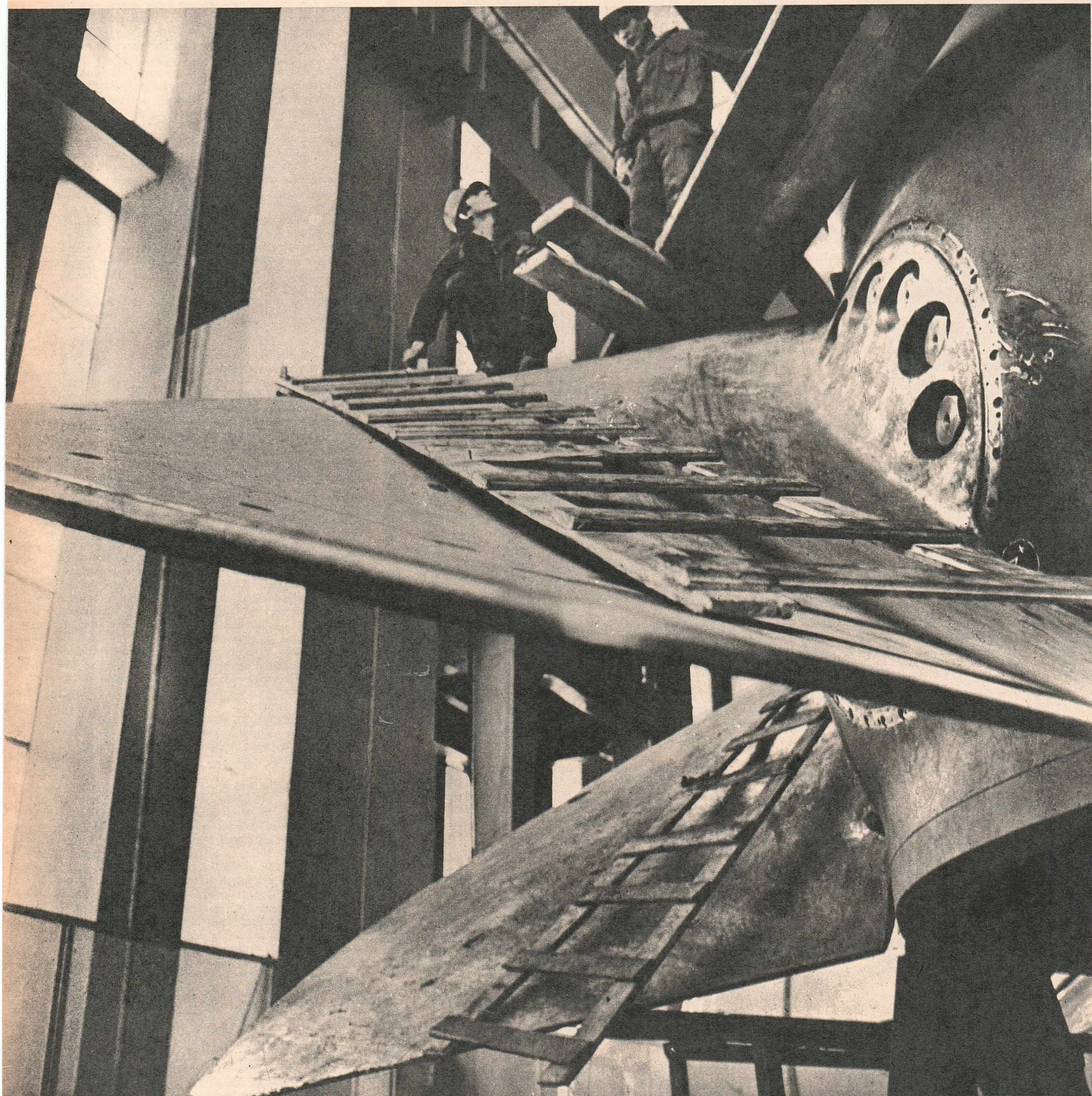
Rotor de turbină menită să stabilească un nou record mondial de putere pentru categoria de turbine căreia îi aparține.
