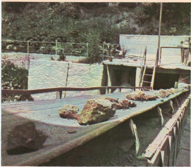
▲ Banda transportoare de calcar către cuptoarele de var.
