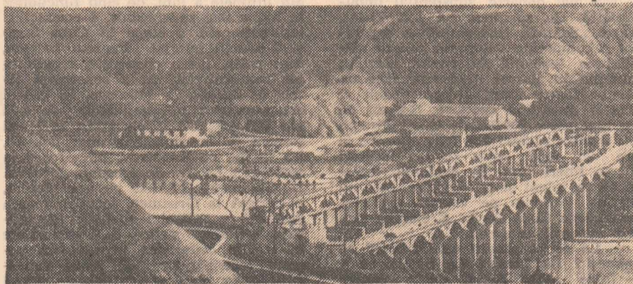
Foto-vedere panoramică asupra centralei hidroelectrice Kanshi de pe riul Miho, construită în R. P. Chineză cu ajutorul populației ținutului Hengtung
