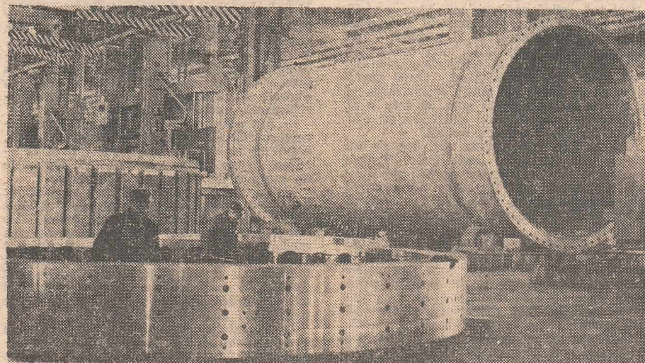
Adevărați coloși de metal, produsele iau drumul beneficiarului după ce, în secția mecano-sudură, și-au încheiat întreaga „cură de slăbire” la care le supun lucrătorii întreprinderii, încă de la proiectare.
