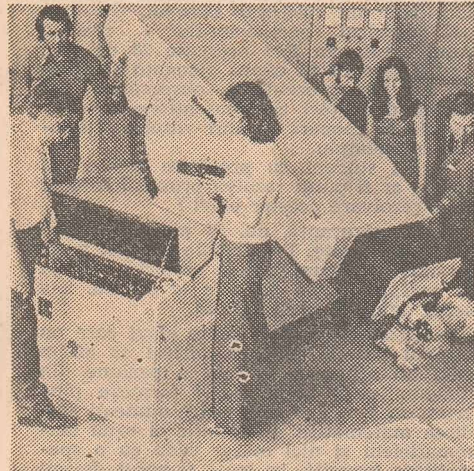
O fotografie document: robotul industrial creat la Facultatea de tehnologie a construcțiilor de mașini de la politehnica bucureșteană, prin colaborarea unui cerc larg de specialiști și de instituții de cercetare. El vestește apariția unei întregi generații de roboți industriali, care, într-un timp nu prea îndepărtat, vor schimba, poate, fața muncii industriale din țara noastră. Proiectul de Directive ale Congresului al XII-lea al Partidului Comunist Român prevede intensificarea cercetărilor în domeniul roboților industriali.
