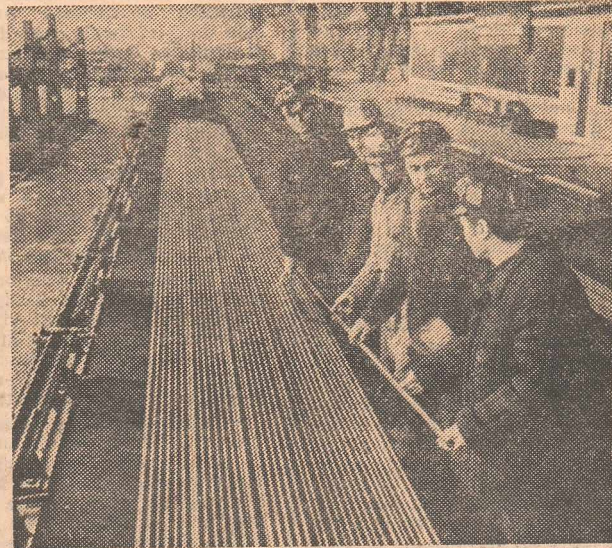
Calitate superioară și productivitate, iată atributele laminorului de țevă inoxidabilă, intrat în funcțiune în primăvara aceasta, la Intreprinderea de țevi REPUBLICA
