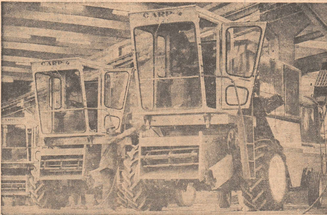
CARP-4, combina autopropulsată pentru recoltaș porumb, o variantă a combinei C-12, destinată, în exclusivitate, recoltării porumbului știuleți. Execută, concomitent, următoarele operații: detașarea știuleților, depănșarea lor, încărcarea lor în remorcă și recuperarea boabelor în buncăr. Datorită ei, în această toamnă, productivitatea recoltării va fi cu 20 la sută mai mare decât în anul trecut
