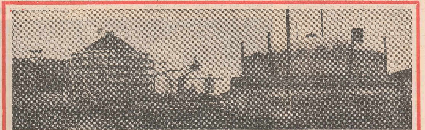
BIOGAZ. Stația de epurare a apelor reziduale ale orașului Tg. Mureș își satisface toate nevoile energetice cu ajutorul biogazului produs. Acest lucru va însemna 200 000 mc de gaz metan economisit. În lucru se găsește proiectul unei sere ce va funcționa cu biogaz. Întreprinderea județeană de gospodărie comunală, folosind biogazul, va fi prima din țară care trece, în funcționarea ei, la utilizarea energiei regenerabile. Aceștia vor fi separate de gunoalele vegetale, vor fi reduse, prin fermentare, iar la o temperatură de 80 de grade devenind neutre pot fi folosite ca îngrășămînt agricol, pentru fertilizarea unor terenuri degradate de pe malul Mureșului, de unde s-a scos balast. Va fi nevoie de acest lucru deoarece în 1981 va începe, prin munca patriotică a organizațiilor Frontului Democrației și Unității Socialiste, a colectivelor care vor primi spre amenajare și folosință, realizarea lucrărilor din al doilea cîntec al Mureșului — Weekend II.
