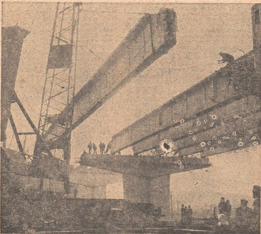
Montarea grinzilor din beton precomprimat de 33 m. lungime având fiecare în parte o greutate de 8 tone
