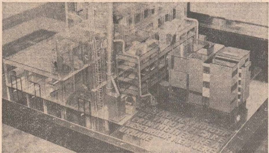
Macheta prototipului instalației de valorificare prin incinerare a deșeurilor menajere.
