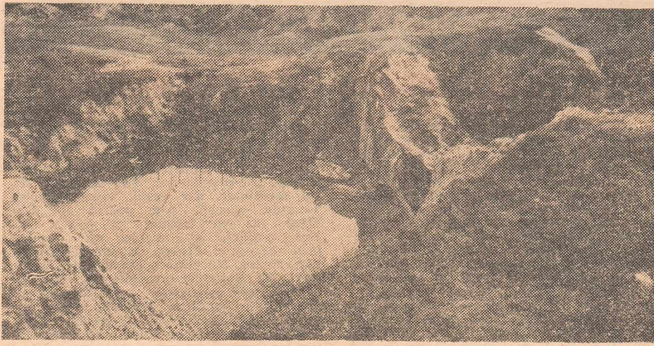
Aci la naștere un lac sărat: Auster, Ocna Sibiului. Procesul de formare are loc, ca să spunem așa, chiar sub ochii noștri.
