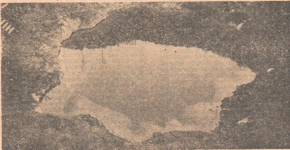
Un strop de cer. (Baia Verde I, Slănic, Prahova).
