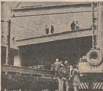
Grinzile, în total vreo 600, au fost preluate de către o macara rutieră direct din vagoanele trenului ce le aducea de la Întreprinderea de prefabricate din Aiud. În timpul ridicării, timp limitat zilnic din cauza traficului la numai trei ore între 10-13, nu trecea nici un tren, iar firele de contact erau scoase de sub tensiune în acest sector.
