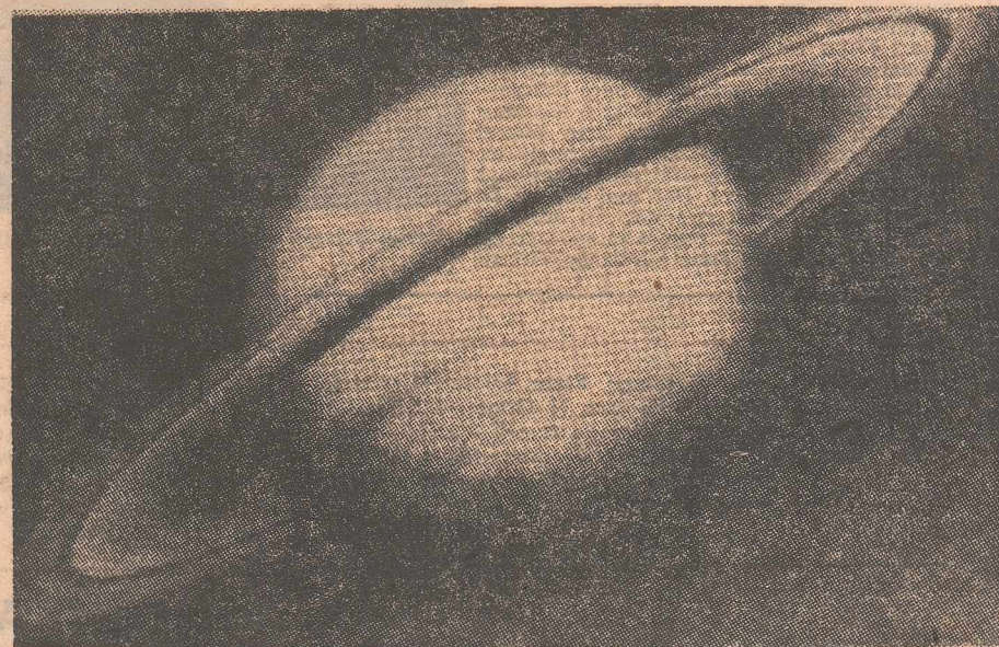
O imagine aproape cunoscută a planetei Saturn, gigantul numărul doi al sistemului solar, și totuși...
