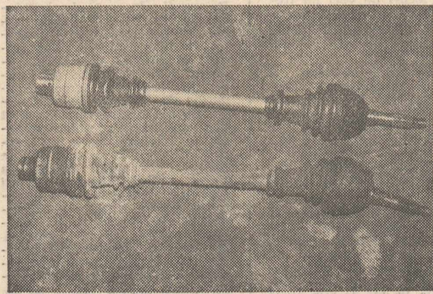
Doi ipostaze ale aceleiași piese: axa planetară (înainte și după operația de recondiționare). Prețul unei piese de schimb noi este de 2100 lei, iar al celei recondiționate de doar 800. Economia de material adusă industriei producătoare: 6,80 kg de oțel special pe bucată. Calitativ, piesa recondiționată este (cel puțin) la fel de bună ca una nouă!
