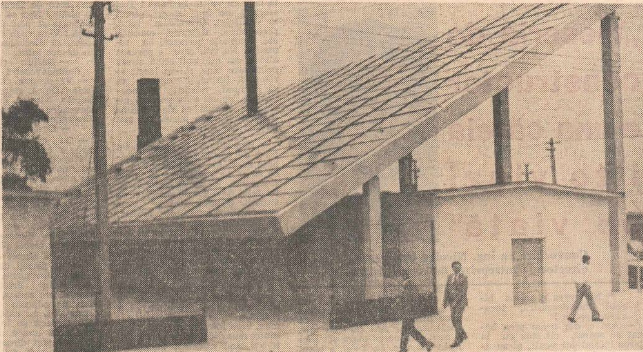
Gratie acestei instalații solare realizată la Stațiunea de cerece tare și producție pomicolă de la Strejești, pot fi deshidratate, într-o singură zi, circa două tone de fructe! Debitul de aer cald e de 4 000 m.c./h, din care aproape jumătate e recirculat.
