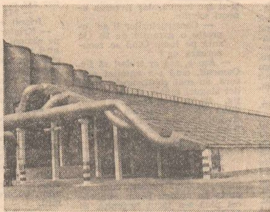
Umiditatea cerealelor se reduce, la Caracal, cu 4 procente pe oră, la un preț de cost (pentru recuperarea investiției) de 53 lei pe tonă de cereale. Operația ar fi costat, dacă s-ar fi folosit motorină, 68 de lei.
