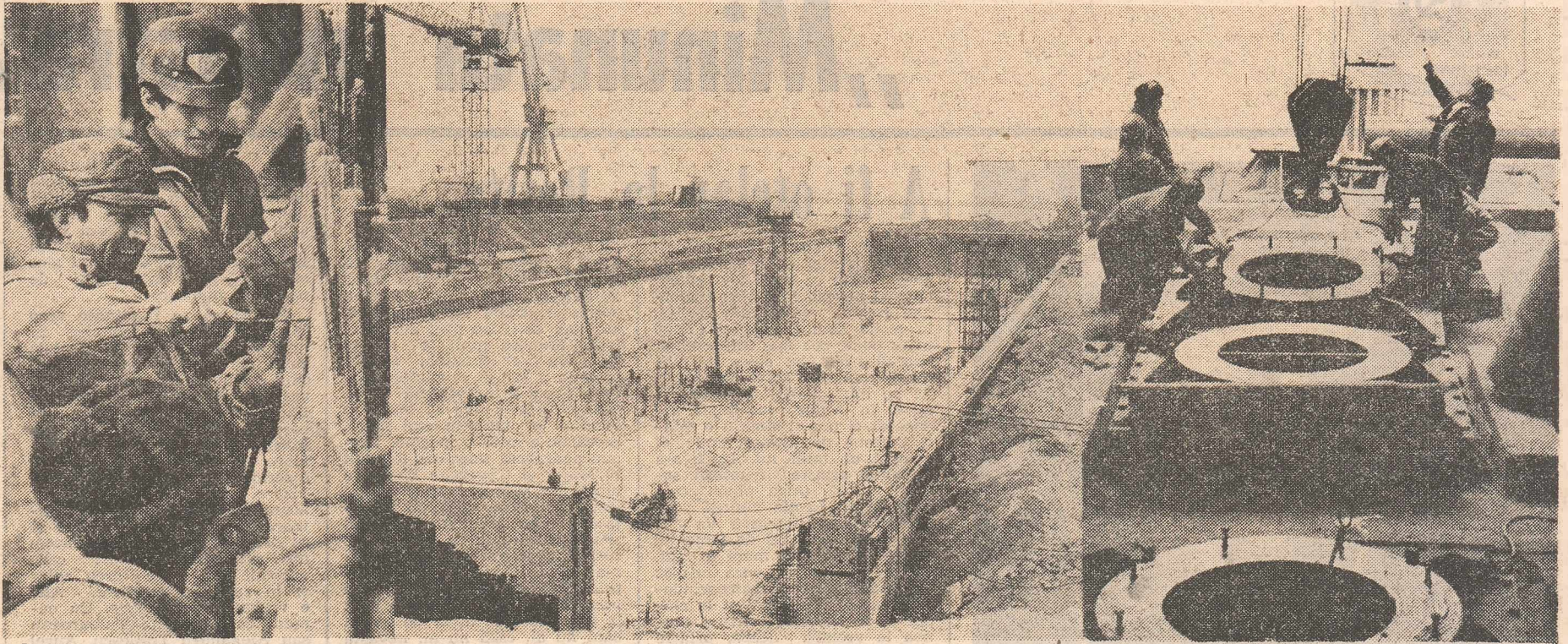
În ansamblul marilor realizări ale litoralului românesc, la Mangalia ia ființă încă un doc uscat pentru repararea navelor de mare tonaj — 150 000 tdw —, lucrare ce se va finaliza într-un timp record, astfel încît primele nave vor intra la reparat încă din acest an.
