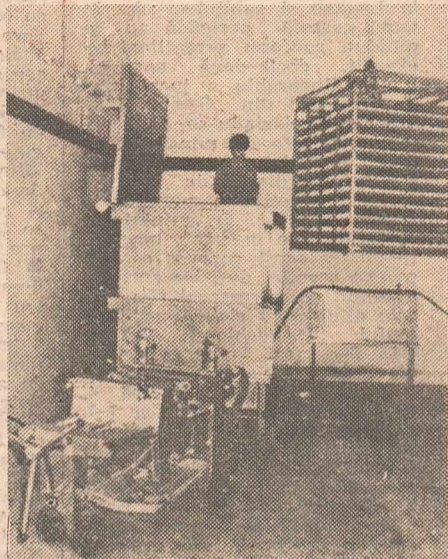
Aparținind inginerului Petru Plăcintă, directorul întreprinderii „Avicola” Bacău, invențiile „Nou procedeu de incubare a ouălor și stație de incubare pentru aplicarea lui” și „Tehnologie nouă de incubare pe principiul totul plin, totul gol”, brevete recent, se remarcă printr-o eficiență economică (numai în unitatea amintită) de ordinul a 7,5 milioane! (stînga).
