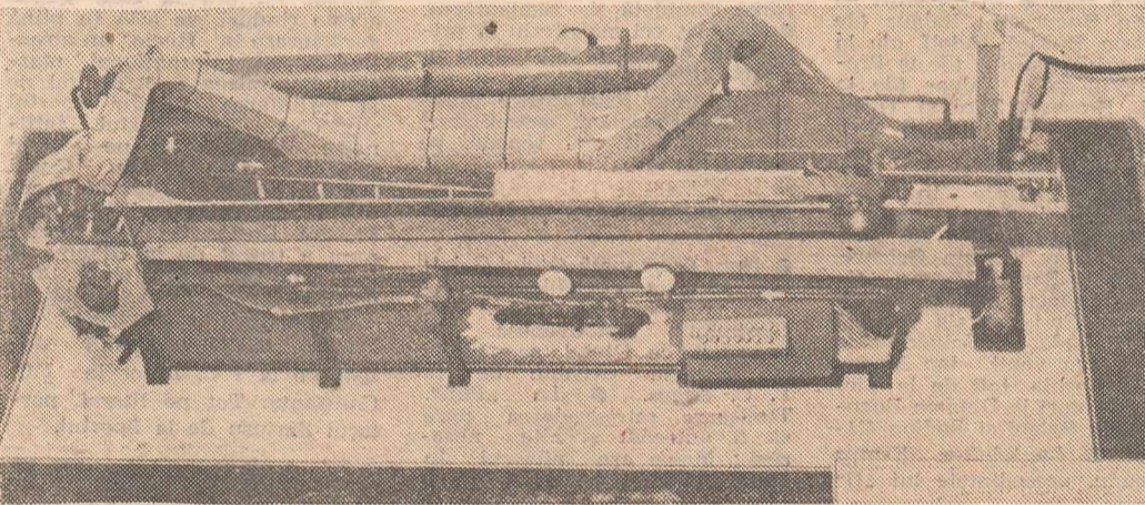
„Mașină pentru recondiționat benzi abrazive”, brevet O.S.I.M. 85 492/1984, autor Ioan Sidor, subinginer la C.P.L. Arad. Aplicată în 13 unități din industria mobilei, ea permite recuperarea benzilor abrazive care, datorită depunerii particulelor de lemn în procesul șlefuirii, erau socotite rebuturi. Autorul, în vîrstă de 42 de ani, ne-a făcut următorul calcul: un metru patrat de pinză abrazivă pe suport de pinză costă în jur de 100 de lei. Noul echipament recondiționează aceeași suprafață cu numai 3,50 lei, fără ca între o bandă inițială și una recondiționată să fie vreo diferență calitativă!
