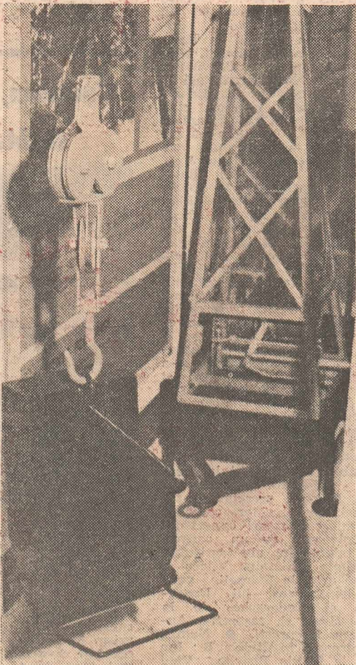
Maistrul Dumitru Rotaru de la I.E.E.L.I.F. Vrancea a pus la punct inovația numită „funicular cu un singur cablu pe remorcă, tractat cu tractorul”. Instalația, ușor de manevrat, poate asigura aprovizionarea cu materiale în locurile foarte accidentate, capacitatea ei de ridicare și transport fiind de 300-100 kg.
