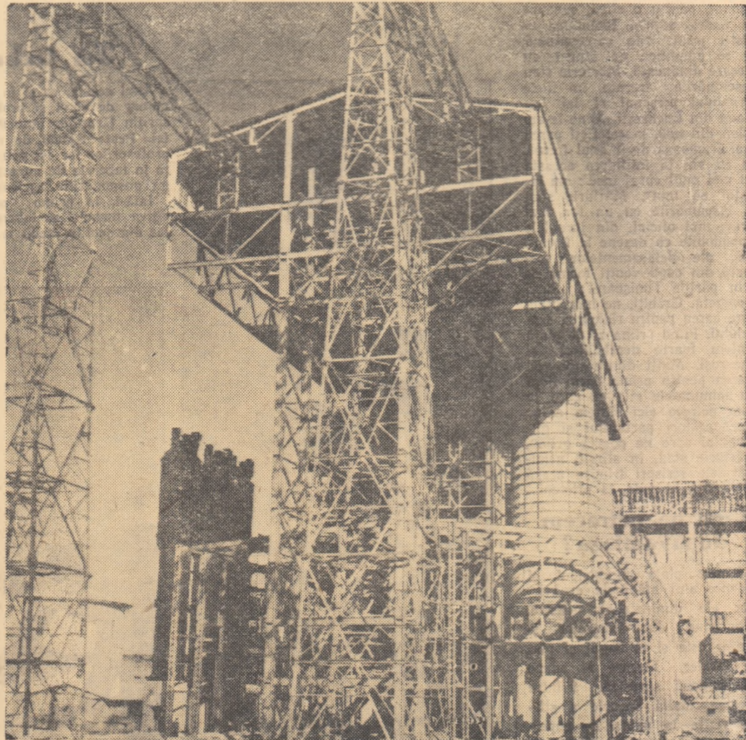
CONSTRUCȚII ALE SOCIALISMULUI: Uzinele de produse sodice de la Govora
