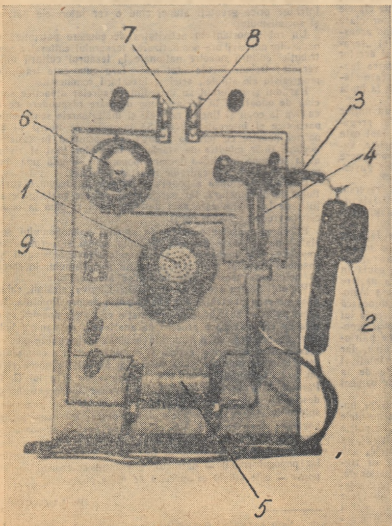
Panou demonstrativ reprezentînd telefonul didactic.
