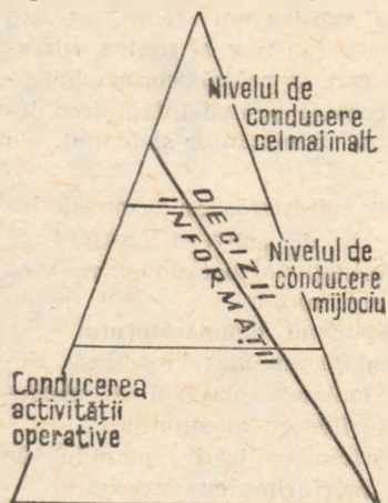
Fig. 1 Piramida informațional-decizională
