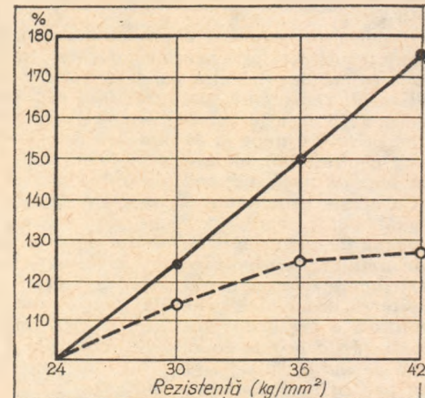
Fig.nr.2. CORELAȚIA DINTRE CREȘTEREA PROCENTUALĂ A REZISTENȚEI MECANICE A OTELURILOR SLAB ALIATE ȘI COSTUL PRODUCȚIEI ACESTORA
