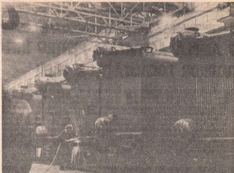
La întreprinderea „Vulcan“ — instalație modernă de fabricație pentru cazanele cu pereți membrană, care se produc pentru prima dată în țara noastră. În imagine: linia de asamblare — flux tehnologic la cazanele de 10 tone/h.
