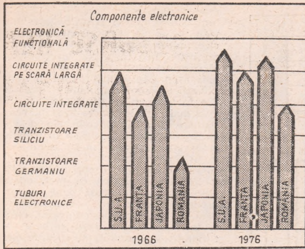
Graficul nr. 1. Dinamica diversificării producției de componente electronice în unele țări.
