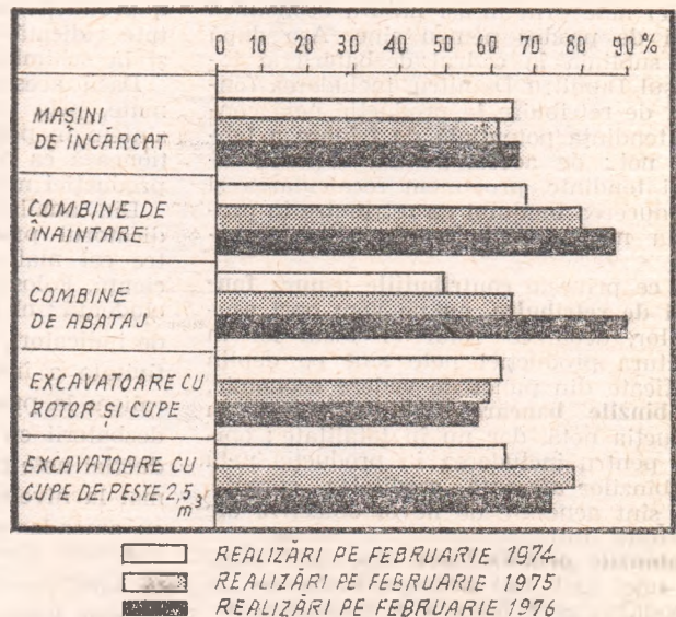
Evoluția gradului de încărcare a fondului de timp disponibil de lucru al unor utilaje de tăiere și încărcare în industria minieră
