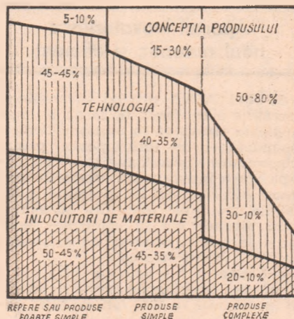
Fig 2. Participarea diferitelor faze la reducerea consumurilor
