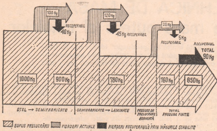
Fig. 1. Pierderile de metal în diferite faze și posibilități de recuperare
