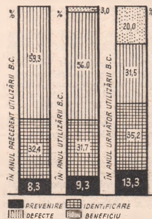
Evoluția costurilor calității prin utilizarea bilanțului calității (B.C.) la întreprinderea mecanică navală din Galați
