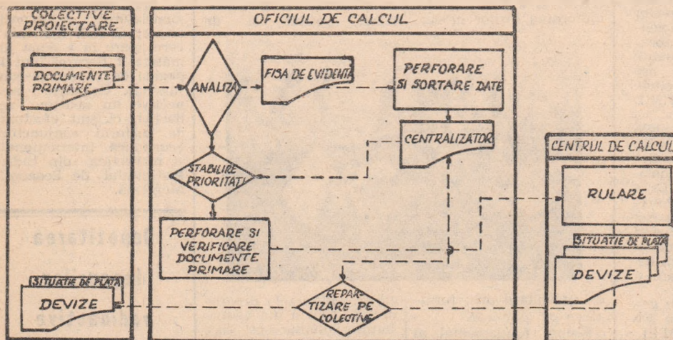
FIG. 2. SISTEM DE CONTROL PENTRU APLICAȚIA DOCEC
