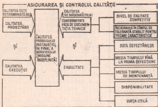
Fig. 3: Fiabilitatea produsului, elementele de cuantificare a acesteia și locul său în problematica de ansamblu a calității.
