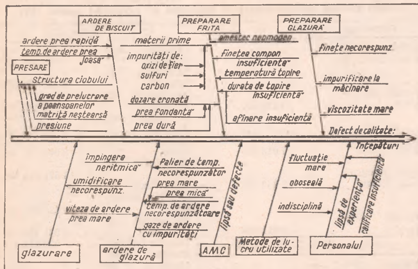
Fig. 4: Diagrama Ishikawa („solz de pește”) a cauzelor și efectelor pentru defectul major la plăcile de faianță — înțepături (pori).
