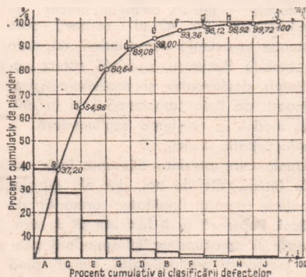
Fig. 1: Diagrama Pareto, construită pe baza analizei statistice a defectelor ce au cauzat pierderi tehnologice la producția de cărămizi GV 29/24.
