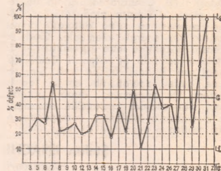
Fig. 2: Diagrama de variație în timp a defectului A. Li — limita inferioară, Ls — limita superioară, C — valoarea centrală (medie).
