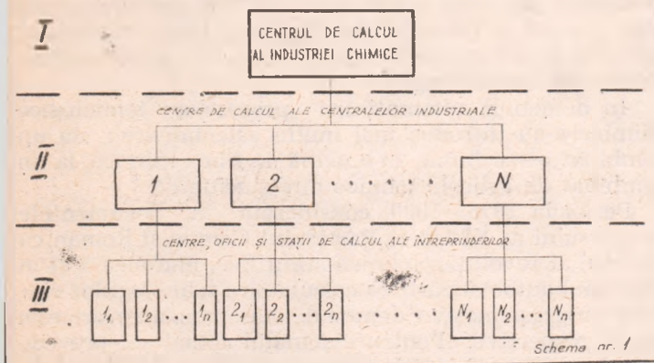
CONFIGURAȚIA GENERALĂ A SISTEMULUI INFORMATIC ÎN INDUSTRIA CHIMICĂ
