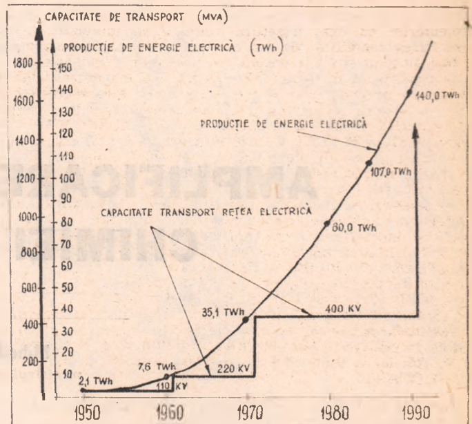
Evoluția producției de energie electrică și a capacităților de transport a rețelei electrice de înaltă tensiune
