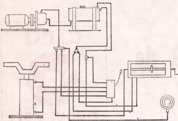
Stand probat sistem frinare auto — S.F.O.A.
