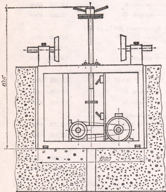
Dispozitiv de depresat anvelope de pe jantă
