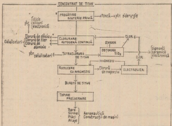
Tehnologie complexă de valorificare integrală cu recirculări active a concentratelor de titan.
