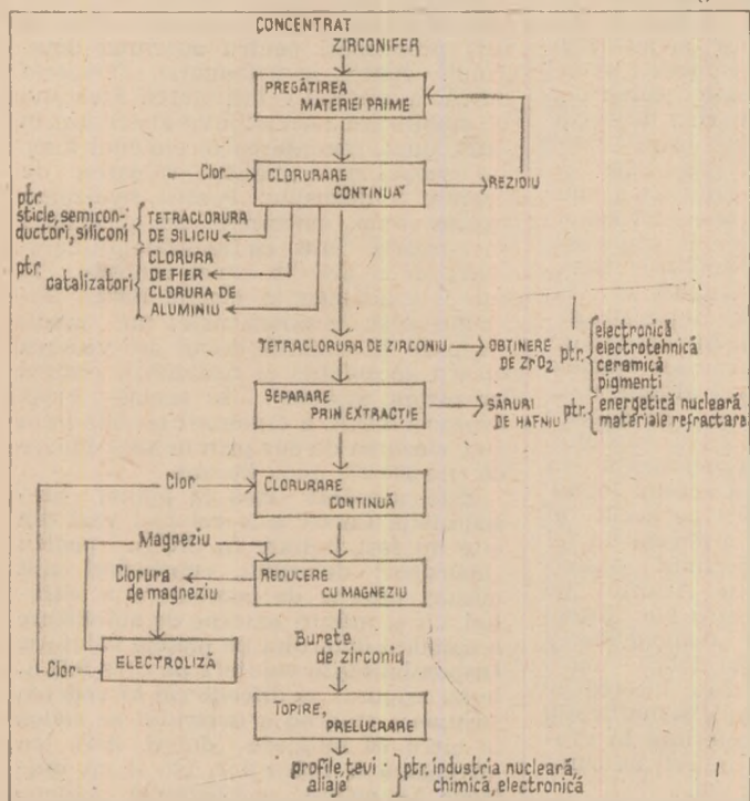
Tehnologie complexă de valorificare integrală cu recirculări active a concentratului zirconifer.
