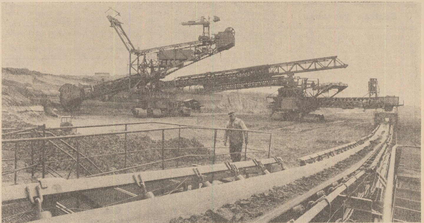
Utilaje de mare randament pentru exploatarea la zi a cărbunelui
