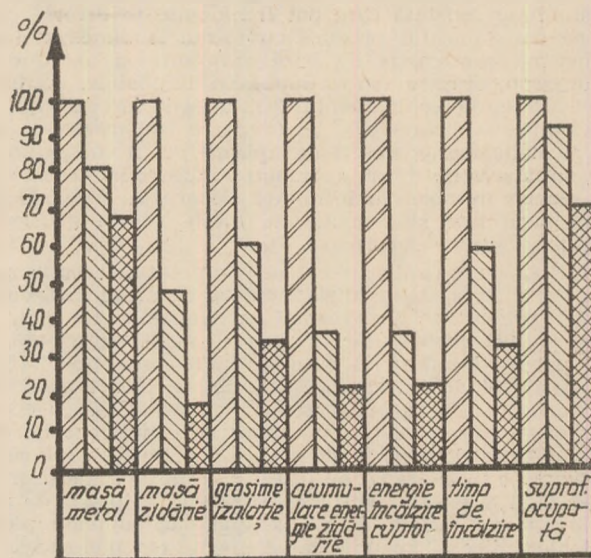
Fig. 2 GRAFIUL REDUCERII UNOR COSTURI PRIN TIPIZAREA CUPTOARELOR INDUSTRIALE
