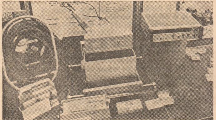
Valorificare practică a licenței Institutului de fizică și inginerie nucleară — aparatul de măsurare a conținutului de cenușă din cărbuni
