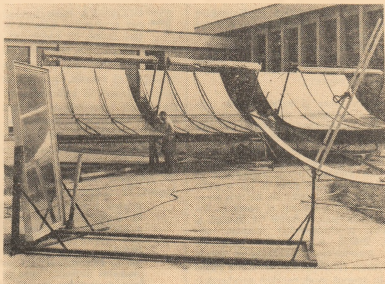
Printre colectivele care desfășoară cercetări în domeniul utilizării energiei solare se numără și cel al catedrei de Termotehnică și mașini termice, de la Facultatea de mecanică a Institutului politehnic București. Instalația de captare din fotografie, realizată la politehnică bucuresteană, este prevăzută cu oglinzi parabolice totalizînd o suprafață de 40 m p.
