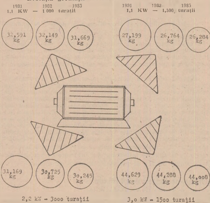
Evoluția greutății motoarelor asincrone în anii
