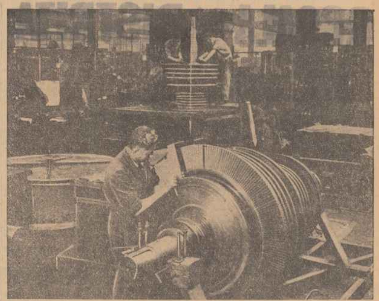
În sectorul turbinelor cu abur de la Combinatul metalurgic Reșița, continuă fabricarea turbinelor de mare putere pentru termocentrale de 4500 KW. Prima serie din aceste agregate este aproape gata pentru planul de export. În clădire: în sectorul rotoare pentru turbine se lucrează la paletele rotoarelor. Foto: AGERPRES
