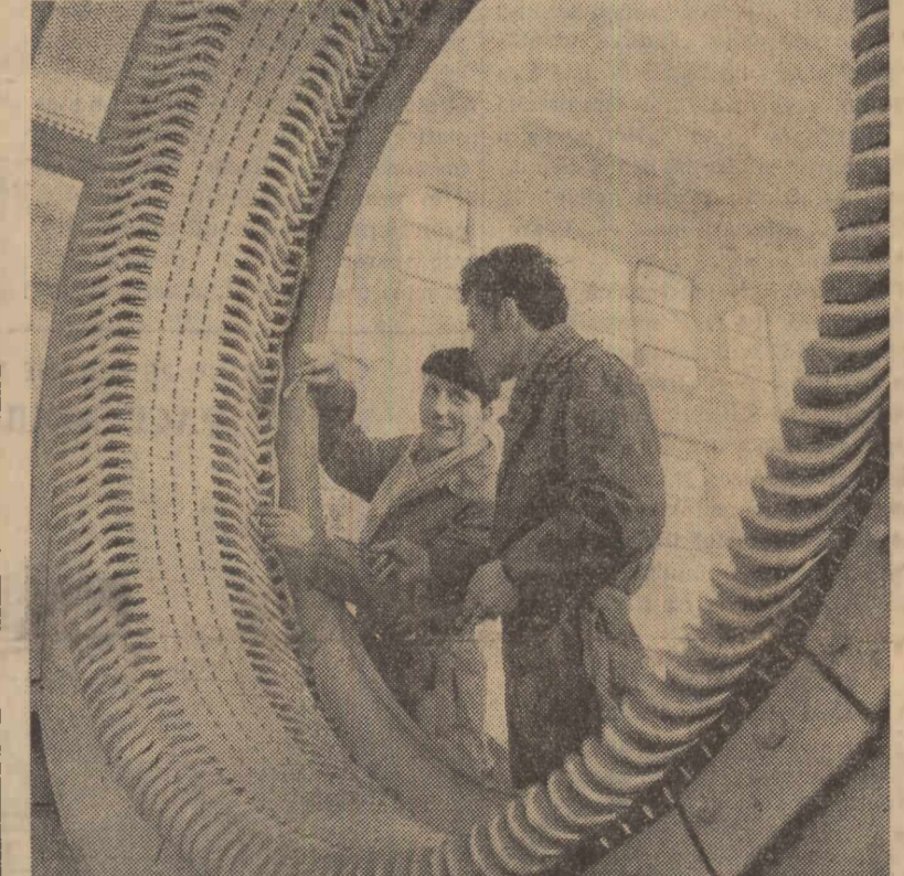
La Combinatul chimic de la Borzești se găsesc în stare de montaj noi instalații și utilaje. În clișeu: înainte de montare se face verificarea statorului și rotorului de la stația centrală de frig Foto: AGERPRES
