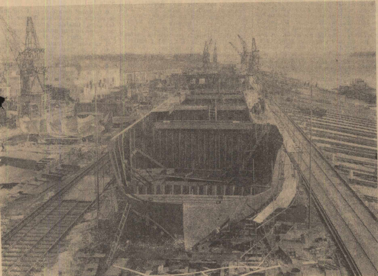
La Santierul Naval Otlenița se construiesc diferite nave maritime și fluviale ca: remorcare, motonave, drăgi cu cuple precum și nave de pasageri. În clișeu: aspect de la asamblarea pe cale a motonavelor de 200 tone
