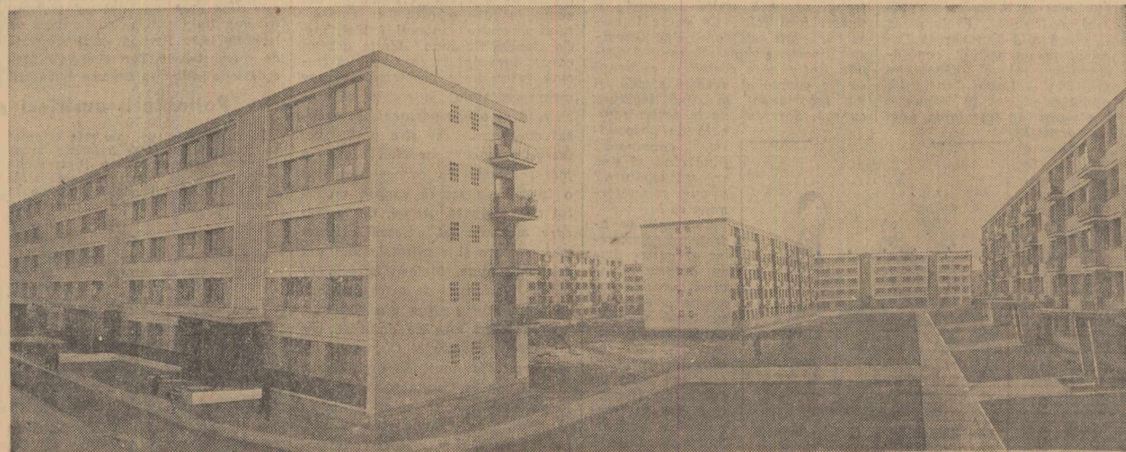
În cartierul Țigîna din Galați se ridică mereu blocuri noi de locuințe. În fotografia noastră se pot vedea cîteva din blocurile recent ridicate din panouri prefabricate și cofraje gîslante.
