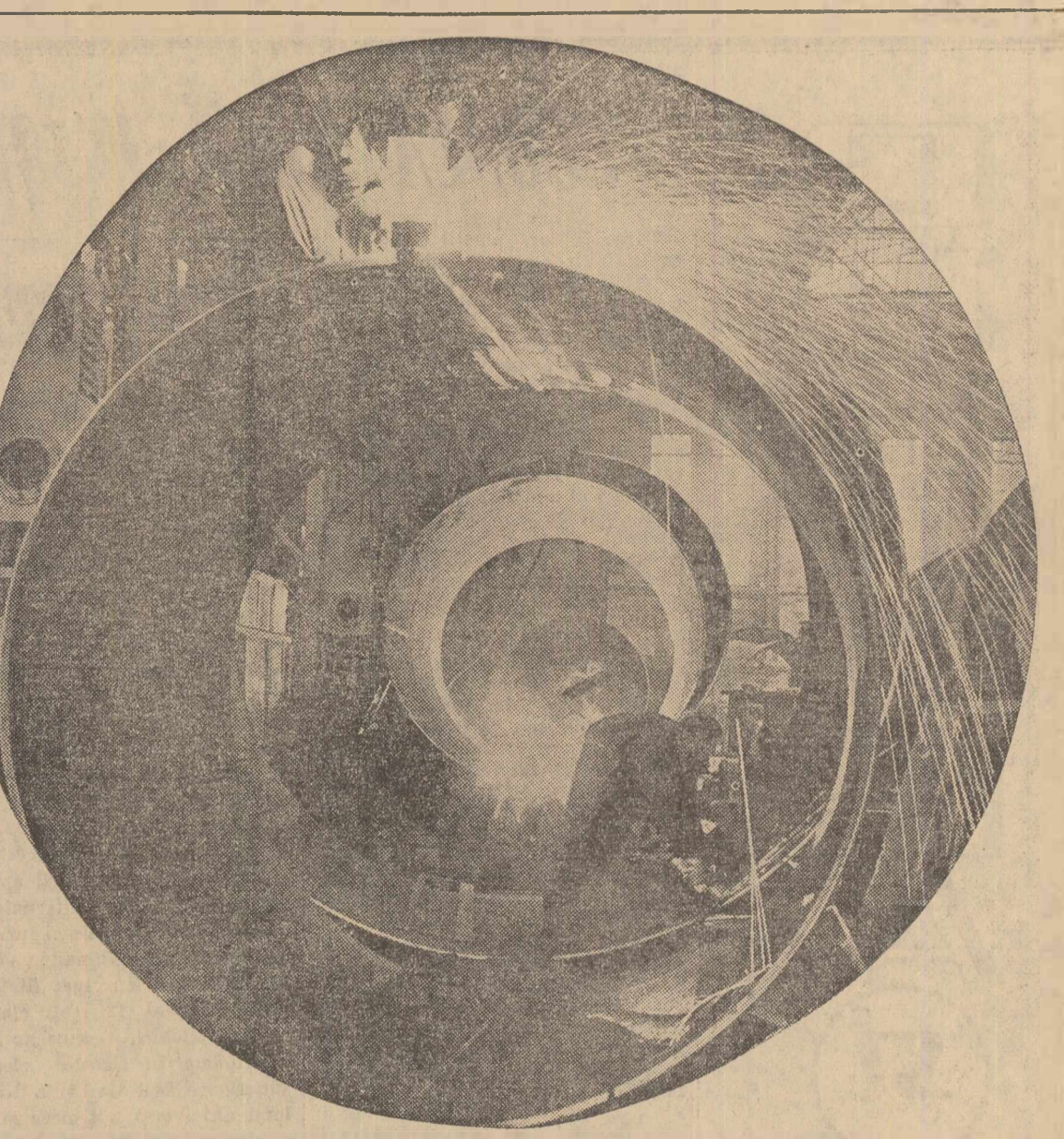
În secția cazangerie a uzinelor „23 August” din București, sudura automată se află într-o permanentă extindere. În cîșeu: Aspect de la sudarea unor virole pentru rezervoare, necesare în industria chimică Foto: AGERPRES
