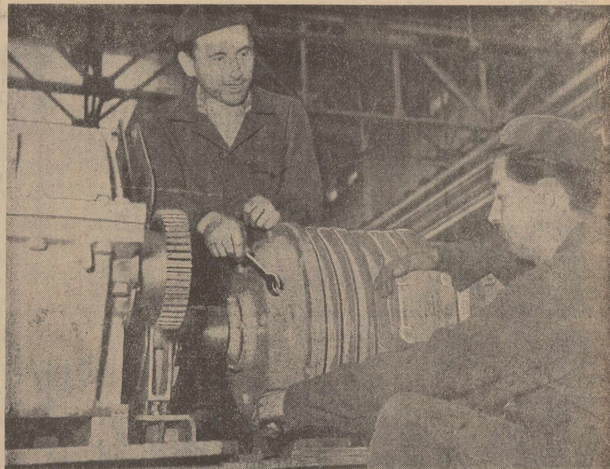
Ioan Mîloș și Nicolae Popil, de la Uzinele mecanice din Timișoara, doi dintre harnicii membri ai brigăzii de pe linia de fabricație a mecanismelor pentru poduri rulante, lucrînd la montajul frînelor.
