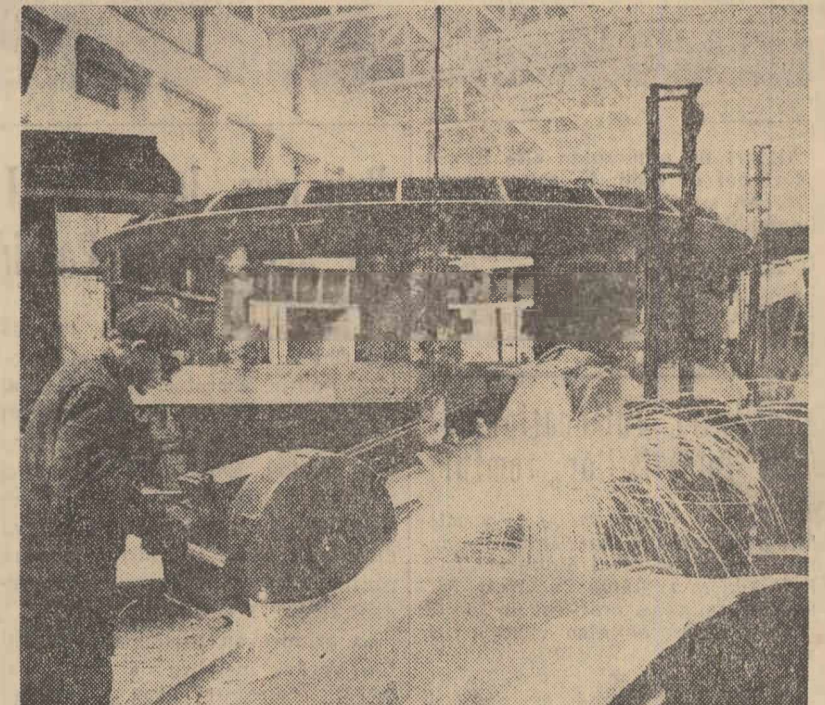
O nouă turbină pentru hidrocentrala de la Bratsk, U.R.S.S. în curs de asamblare la uzinele „Cel de-al XXII-lea Congres al P.C.U.S.”
